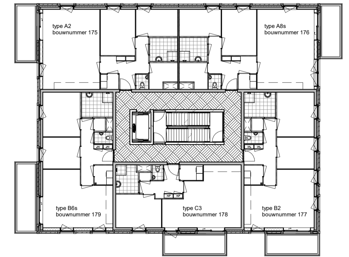
vierde verdieping
