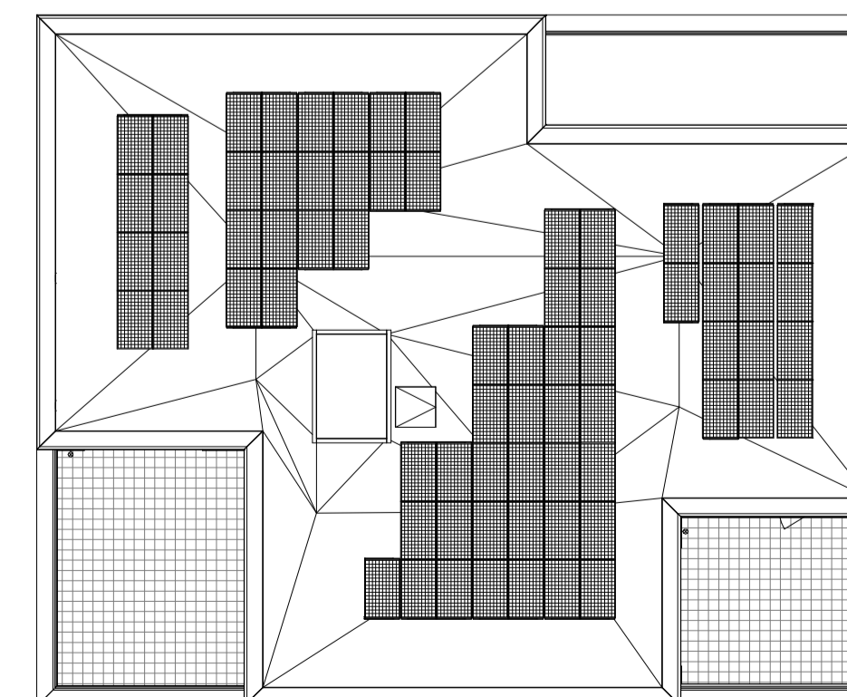
dak
