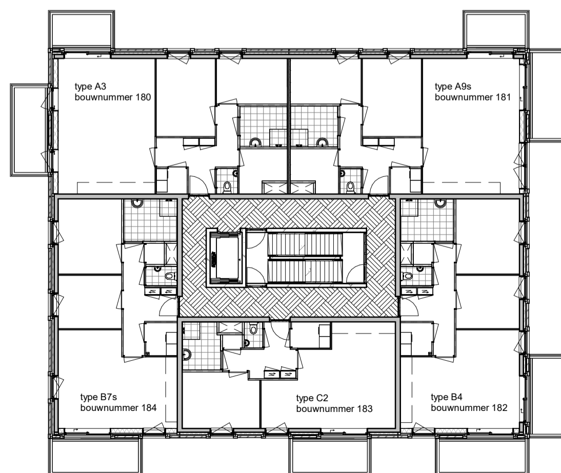
vijfde verdieping
